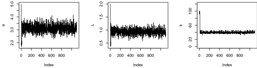
Figura 8.2: Cadeias geradas para os parâmetros \theta , \lambda e k .
