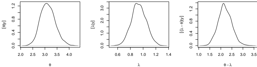
Figura 8.4: Posteriors de \theta , \lambda e de (\theta - \lambda) .
