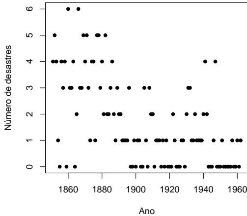
Figura 8.1: Números de desastres por ano em minas de carvão.
