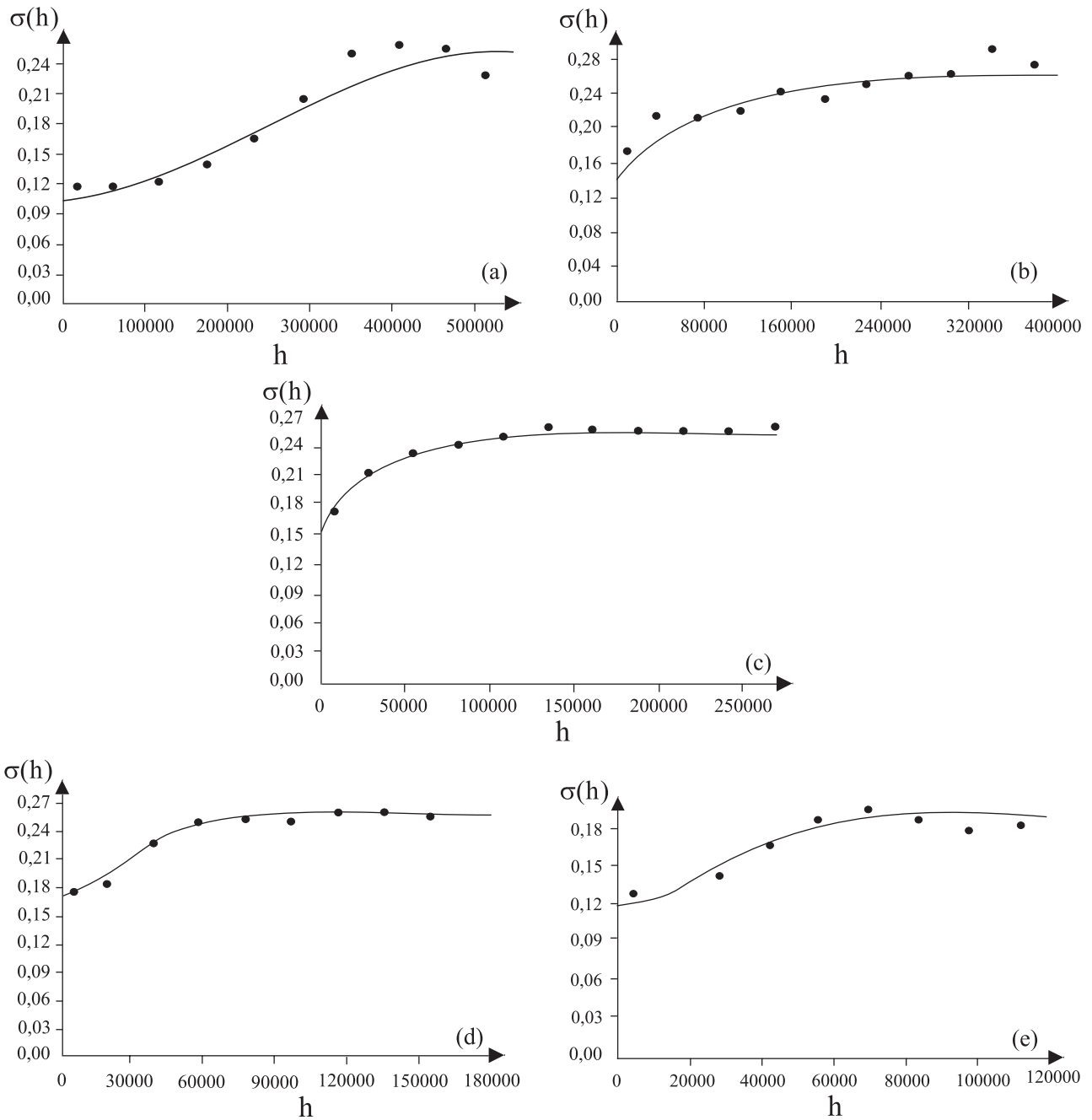
Figura 1. Variogramas dos cinco cortes da variável alumínio: (a) q_{0,2} = 0,6 ; (b) q_{0,4} = 2,19 ; (c) q_{0,5} = 2,90 ; (d) q_{0,6} = 3,80 ; (e) q_{0,8} = 5,40 .
